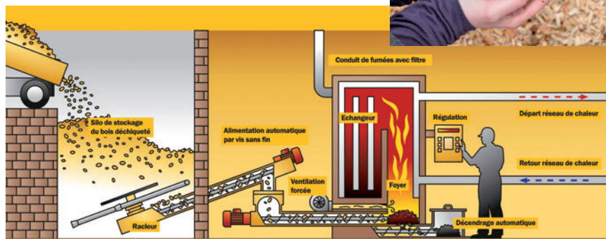
Principe de fonctionnement Future chaufferie
